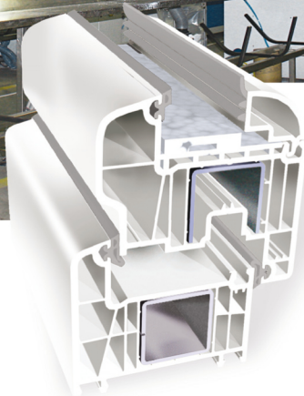
Profil półzlicowany
